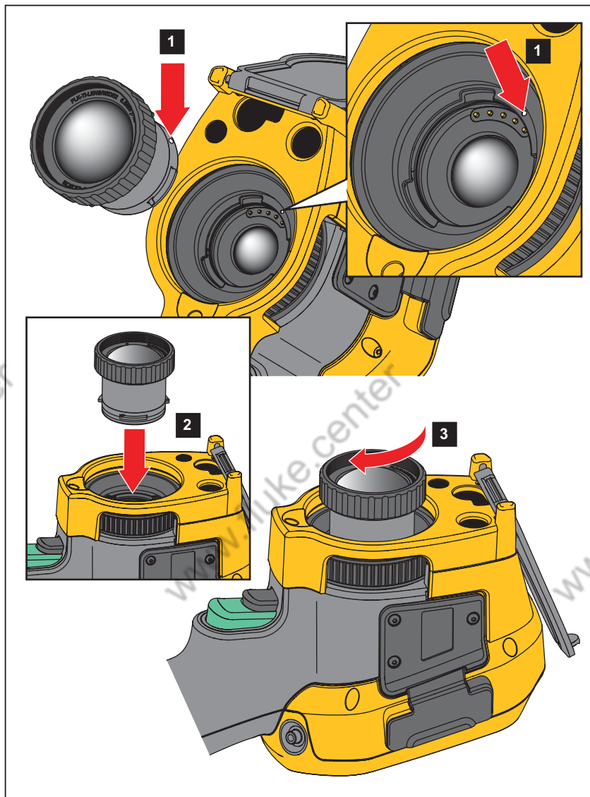
Рисунке 1. Установка дополнительного объектива
