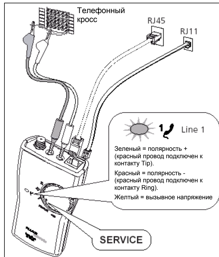
Рисунок 2. Проверка телефонных линий и полярности.
