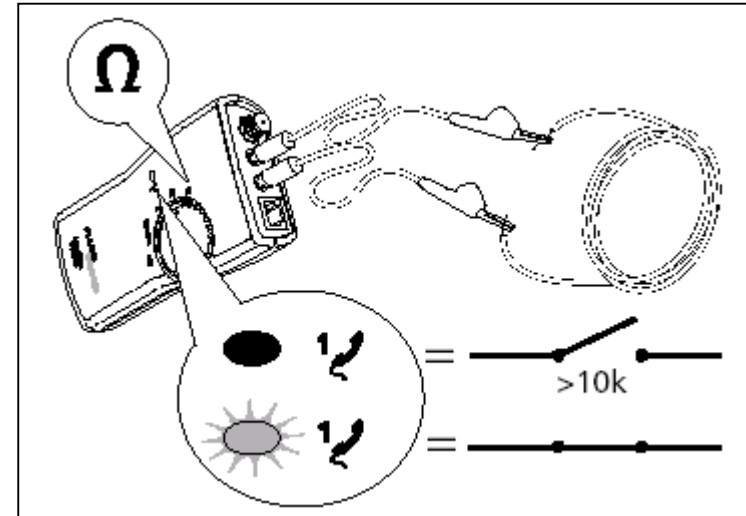
Рисунок 3. Тестирование непрерывности
