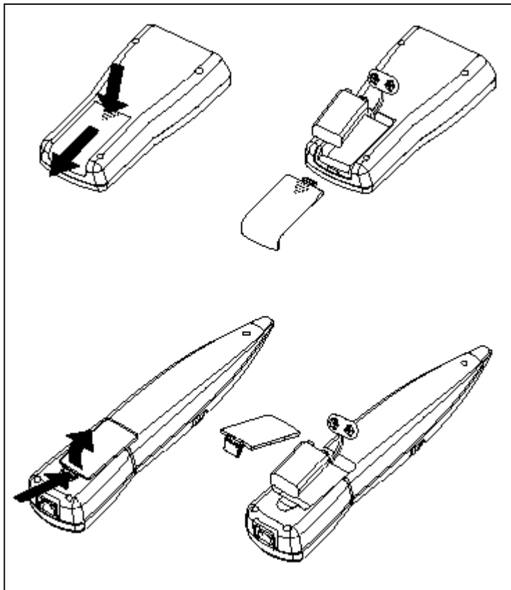
Рисунок 5. Замена батареи
