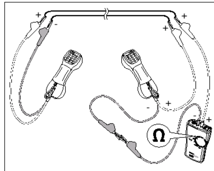
Рисунок 4. подача питания комплекту оборудования для тестирования телефонии
