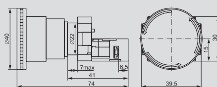
Габаритные размеры
