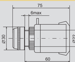
Габаритные размеры
