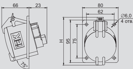
Стационарные розетки для скрытой проводки ССИ-423÷ССИ-425
