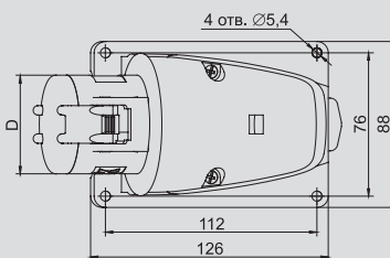
Стационарные розетки для скрытой проводки ССИ-423÷ССИ-425
