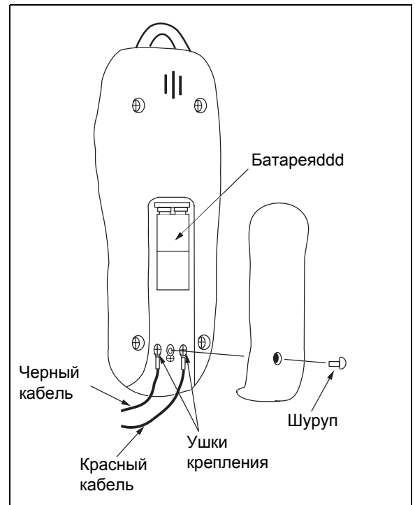
Рис. 3. Замена батареи и кабеля для подключения к линии
