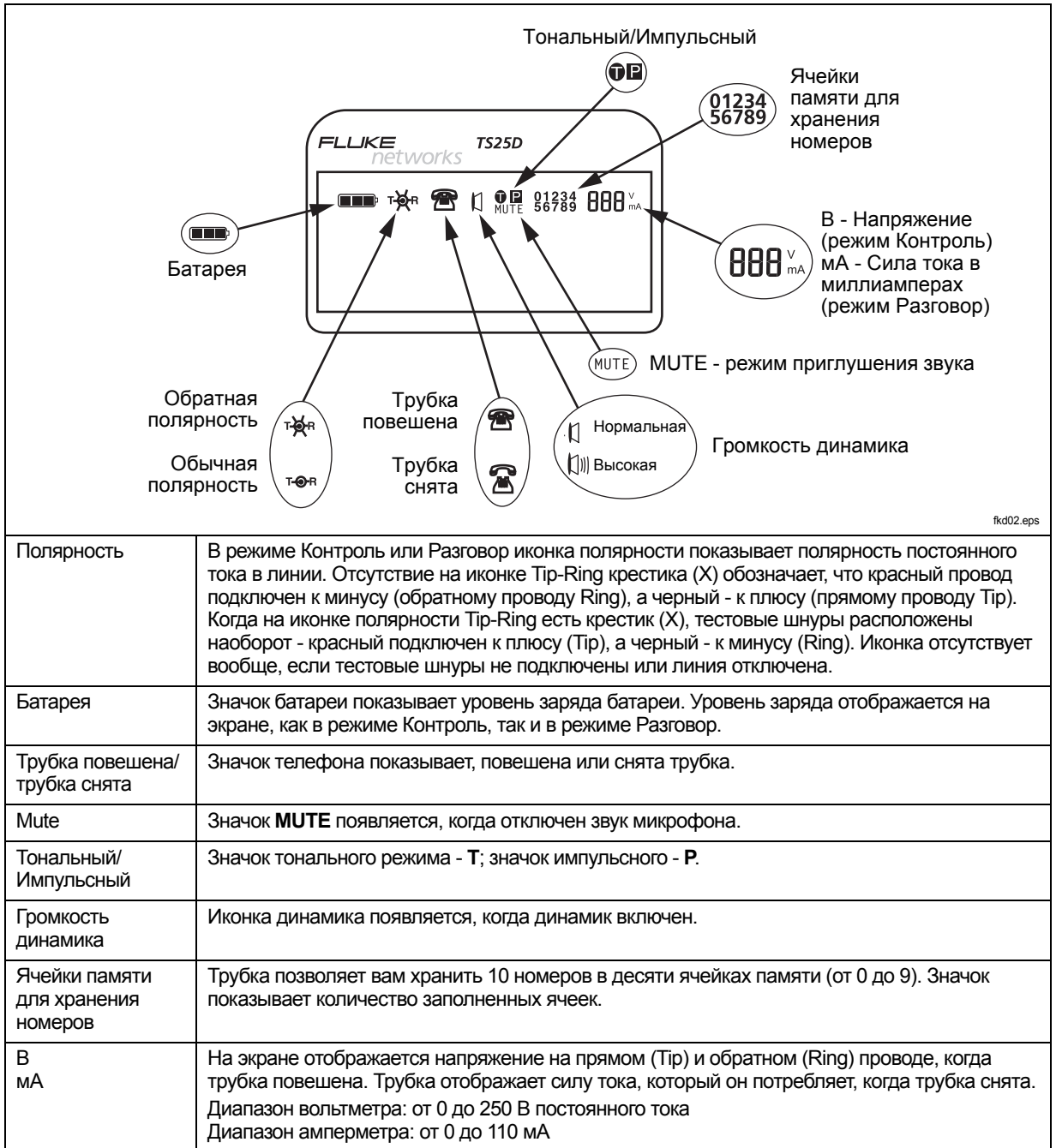
Рис. 2. Иконки на дисплее тестера TS25D
