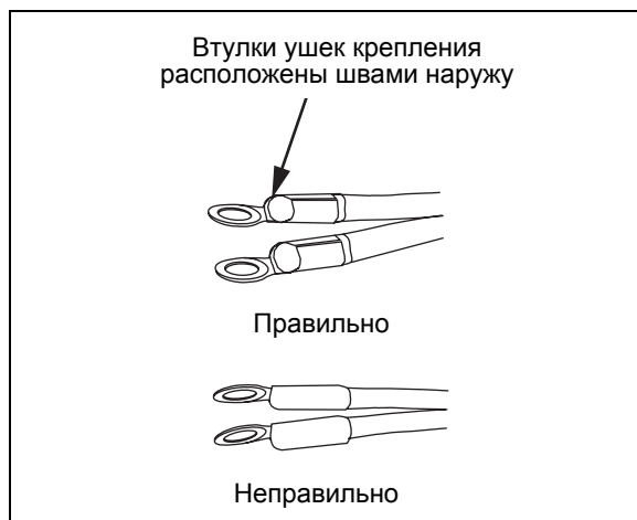
Рис. 4. Положение ушек крепления тестового шнура
