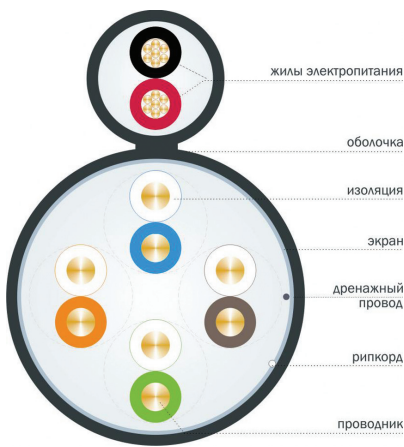
Вид кабеля в поперечном разрезе
