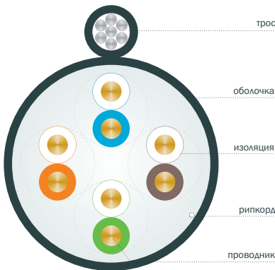
Вид кабеля в поперечном разрезе
