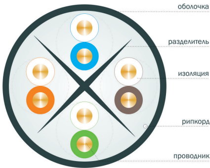
Вид кабеля в поперечном разрезе
