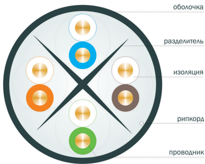
Вид кабеля в поперечном разрезе
