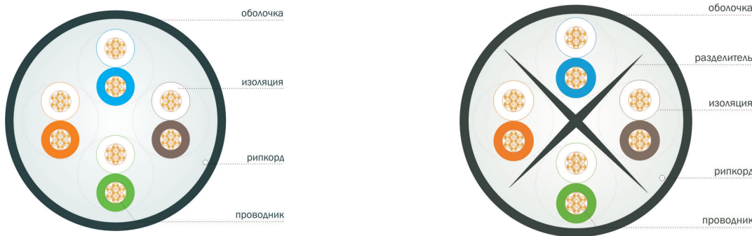
Вид кабеля в поперечном разрезе
