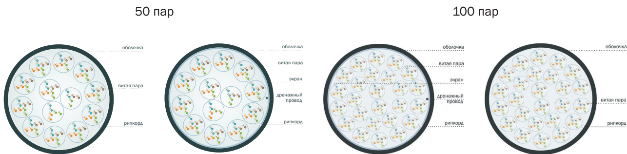
Вид кабеля в поперечном разрезе
