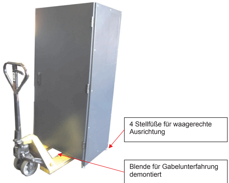
Abbildung: Transport mittels Hubwagen
