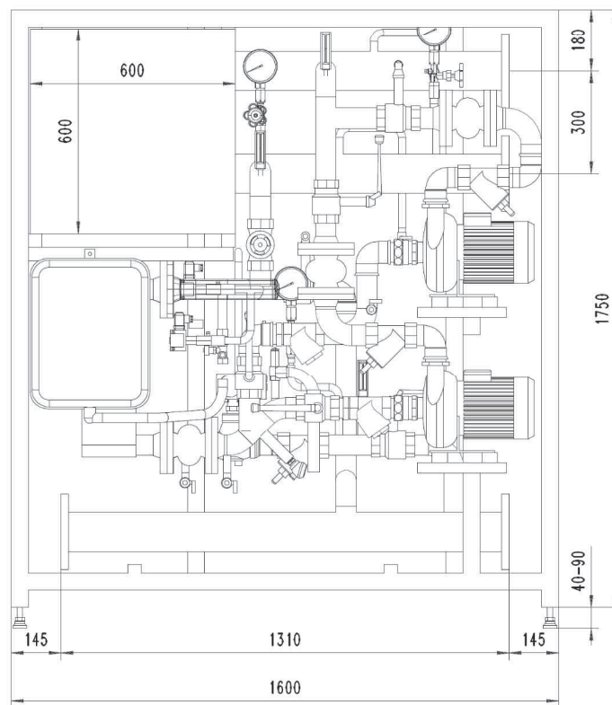
Abbildung CoolTrans 100 (Standard) Ansicht von vorn
