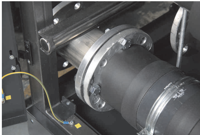
Abbildung: Flanschverbindung, hier Zwischenflansch für Anschluss einer weiteren CTU
