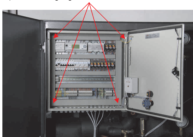
Abbildung: Befestigungsschrauben Schaltschrank
