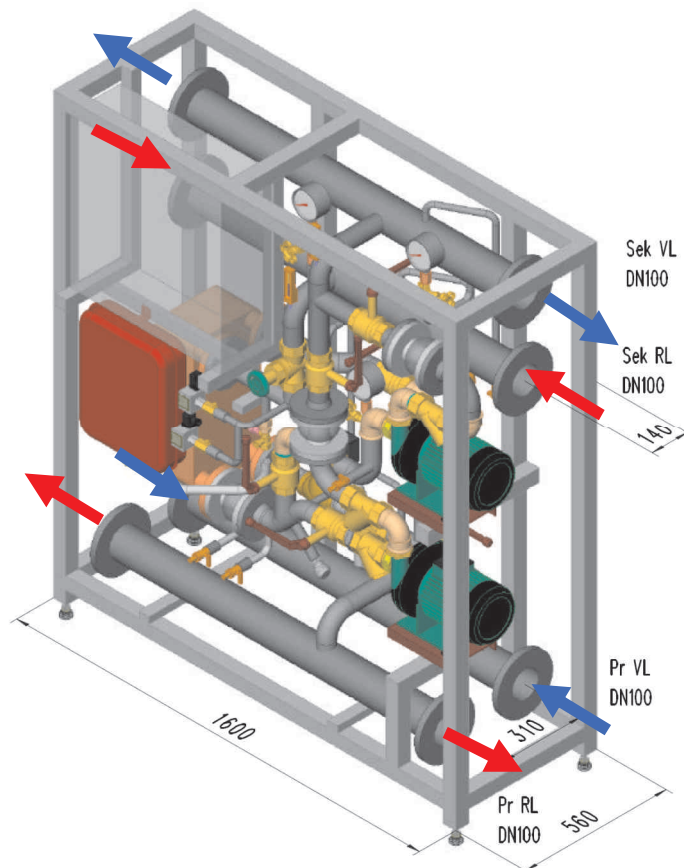
Abbildung CoolTrans 100(3D))
