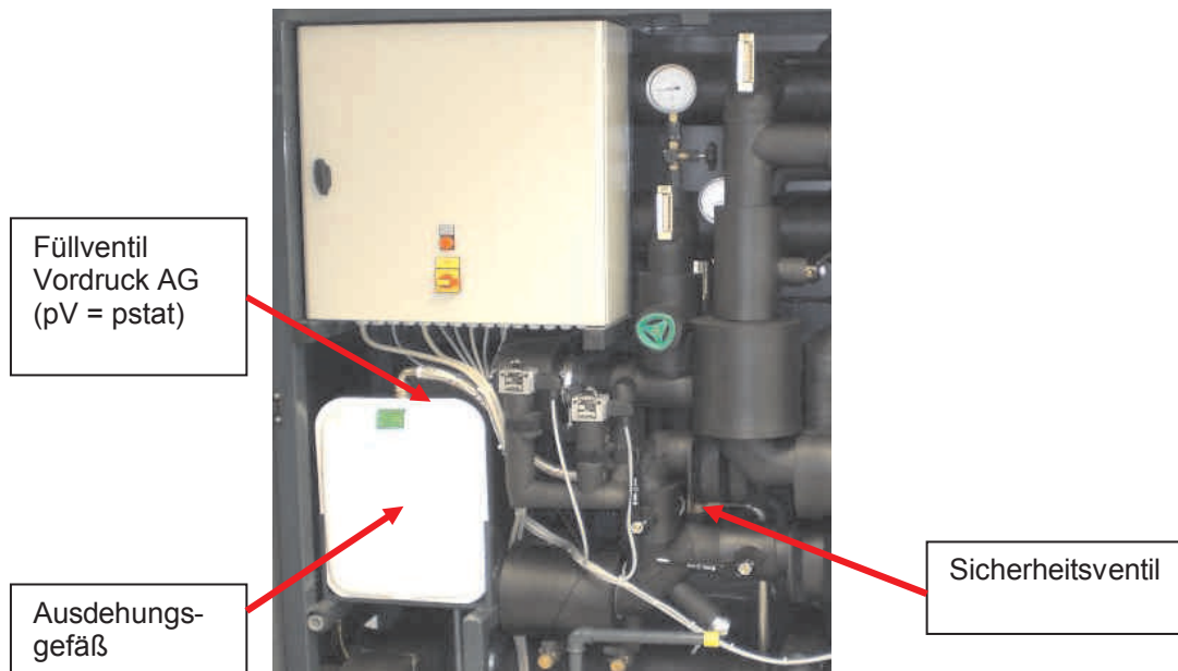
Abbildung: Sicherheitsbaugruppe
